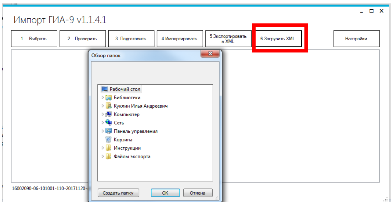
Рисунок 18. Загрузка XML-файла
