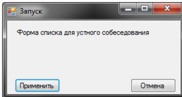
Рисунок 9. Настройка параметра
