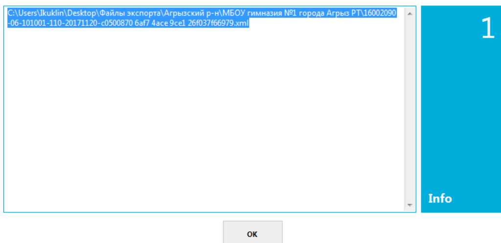
Рисунок 19. Успешная загрузка
